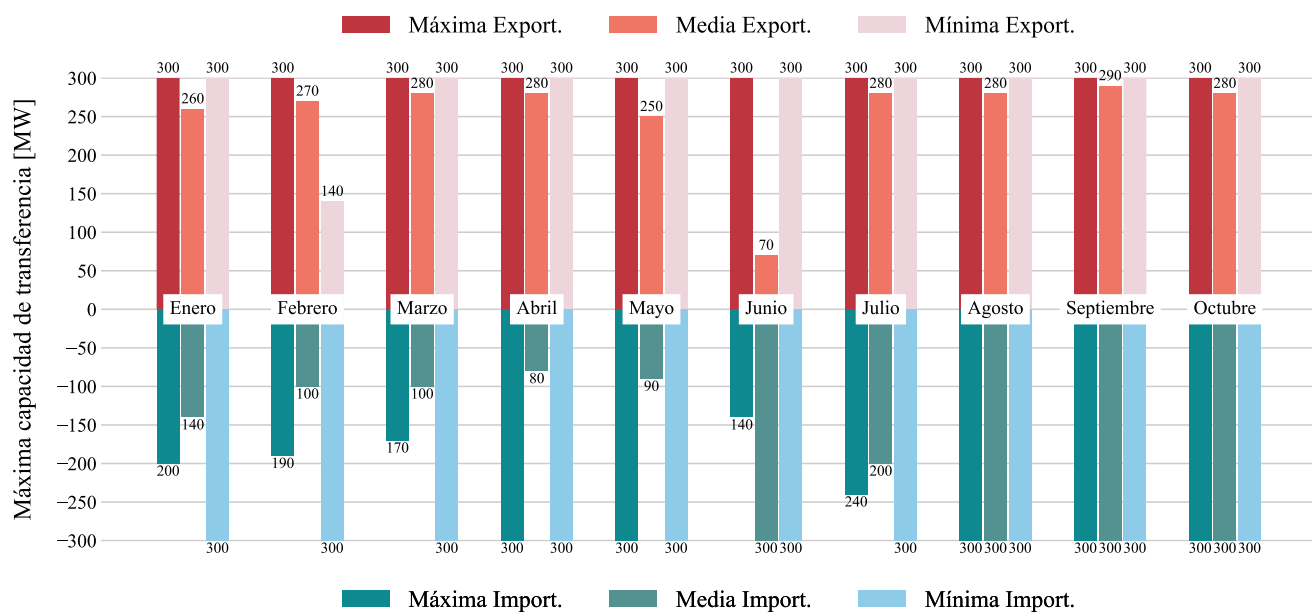
Figura 4. Máxima Capacidad de transferencia con Guatemala para 2025
