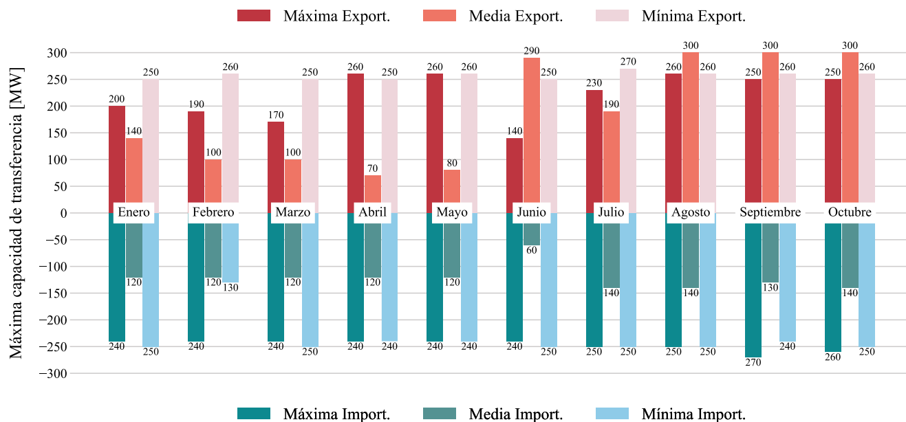
Figura 8. Máxima Capacidad de transferencia con Nicaragua para 2025
