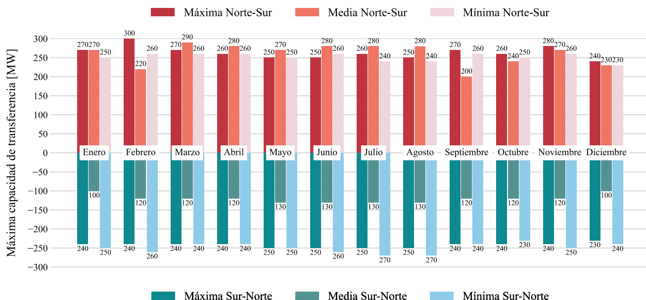
Figura 1. Máxima Capacidad de Porteo para 2024
