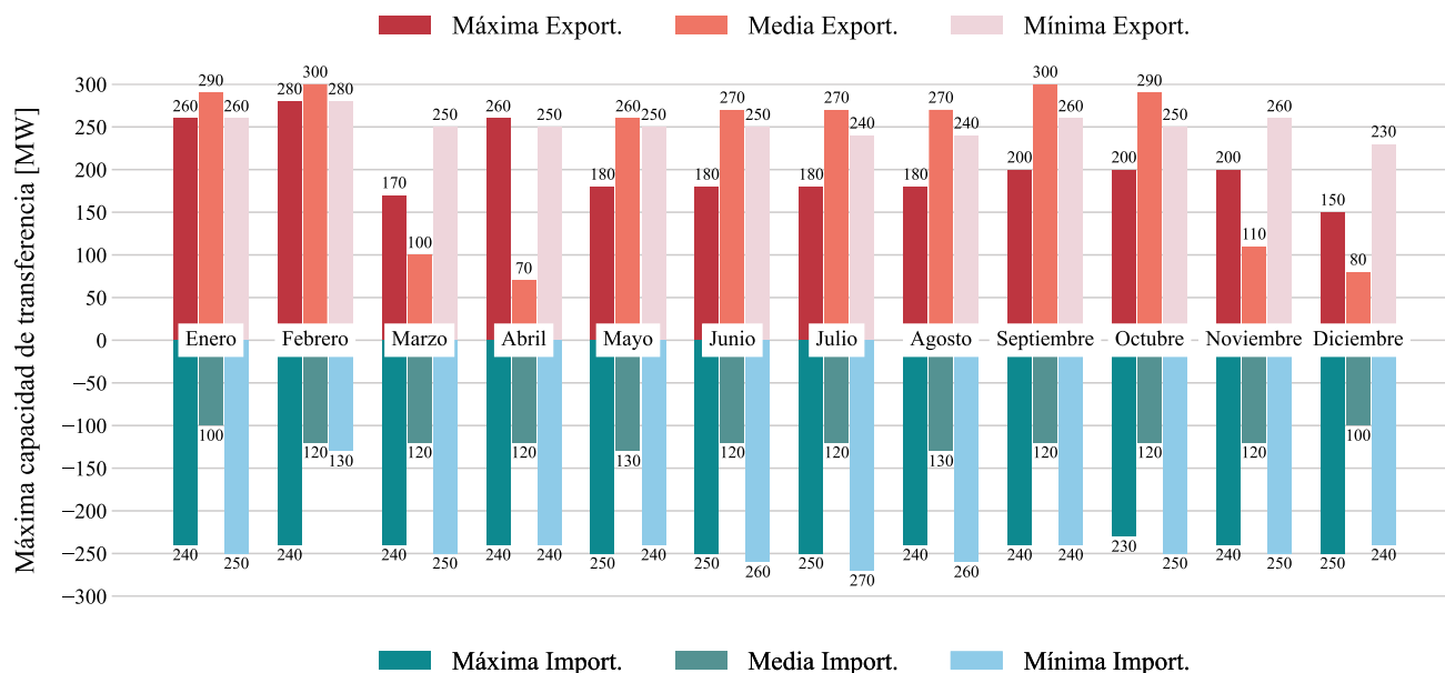
Figura 7. Máxima Capacidad de transferencia con Nicaragua para 2024
