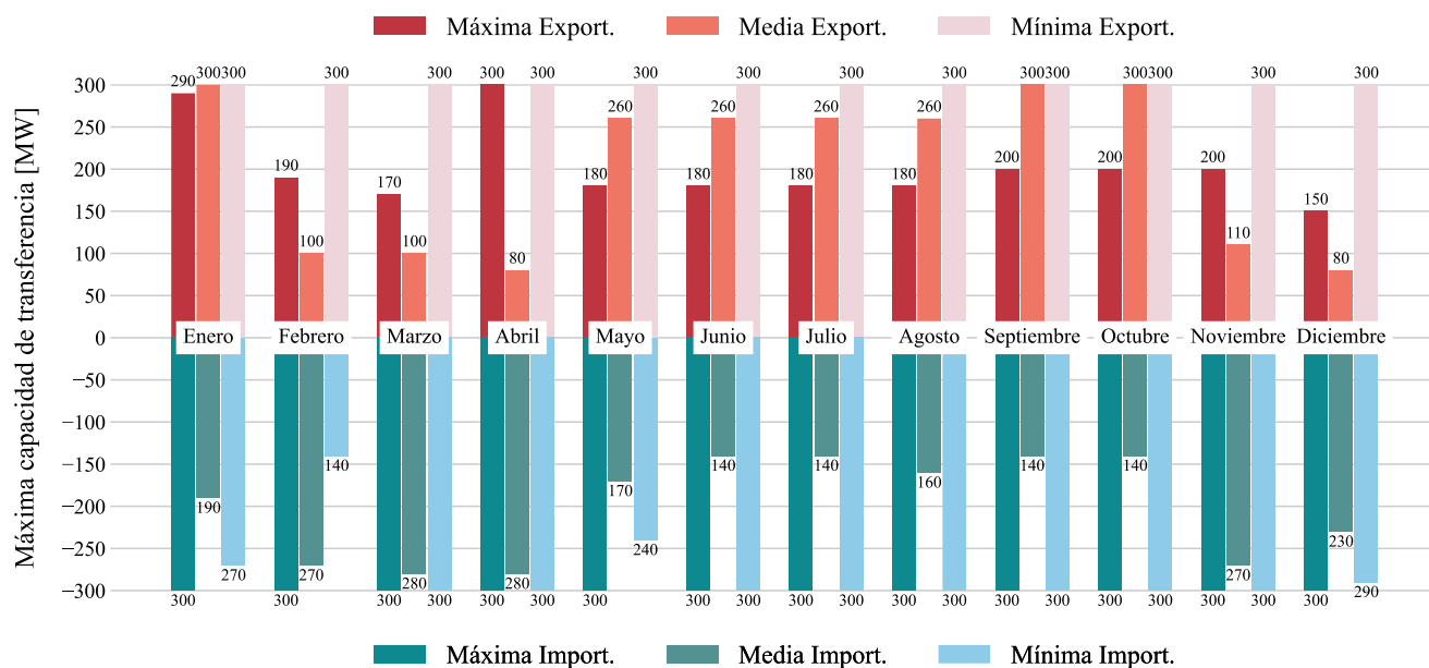
Figura 3. Máxima Capacidad de transferencia con Guatemala para 2024
