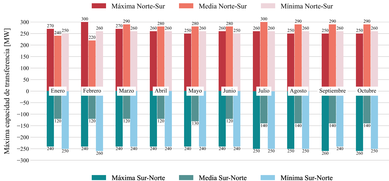
Figura 2. Máxima Capacidad de Porteo para 2025
